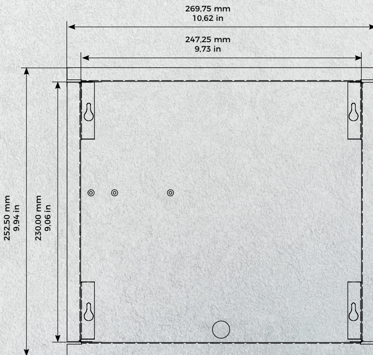
Boîtier de montage arrière (encastré)
